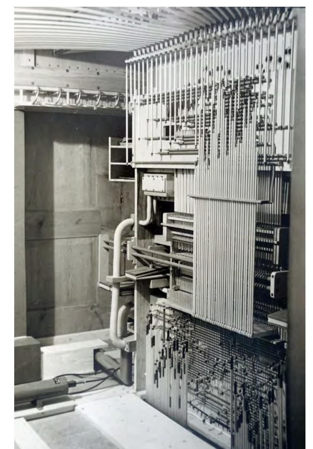
Umbau 1954. Rückansicht des Spieltisches und Traktur (Übertragungssystem)
