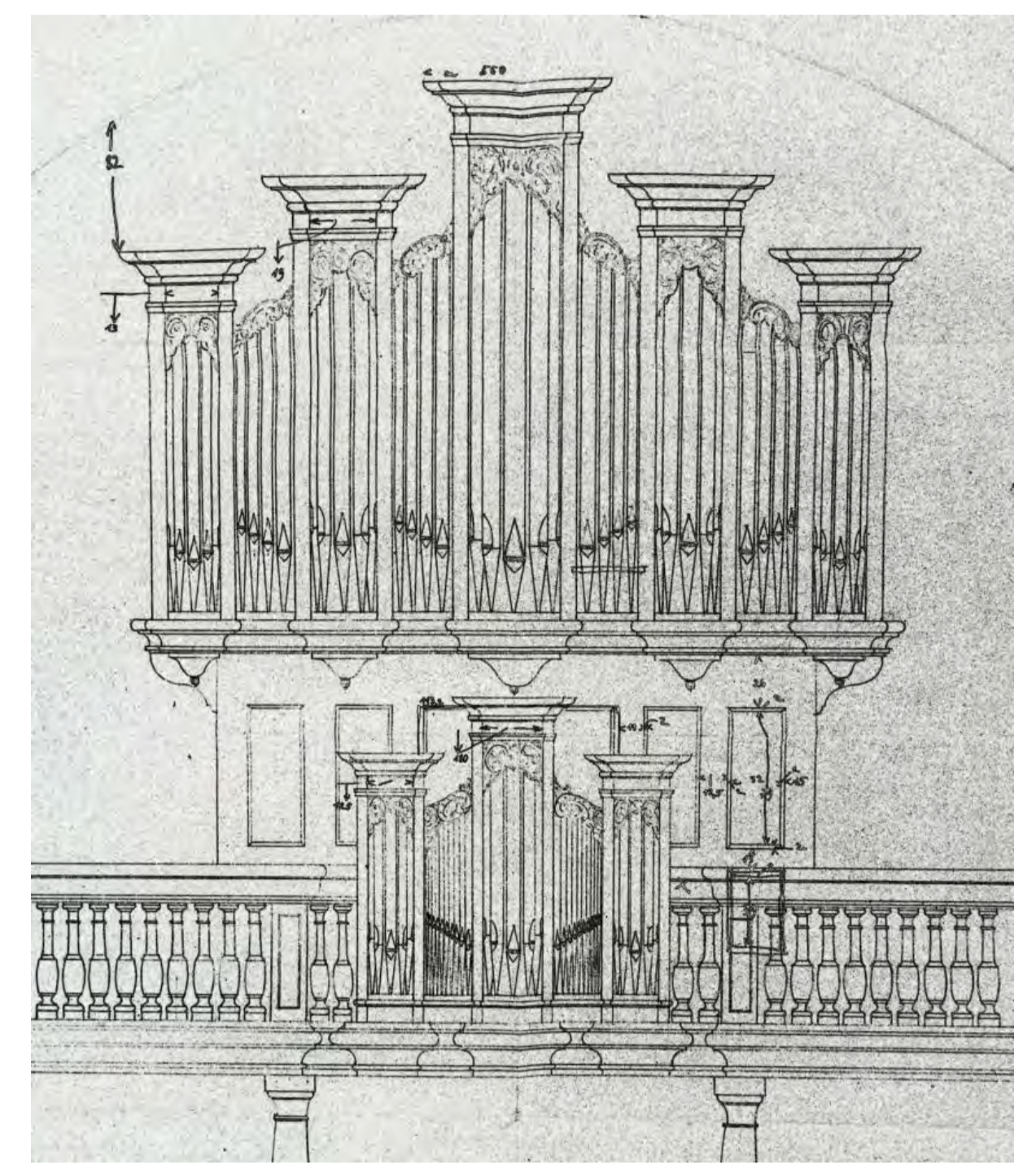
Vorderansicht des Orgelprojektes 1953 mit Massangaben von Ernst Schiess
