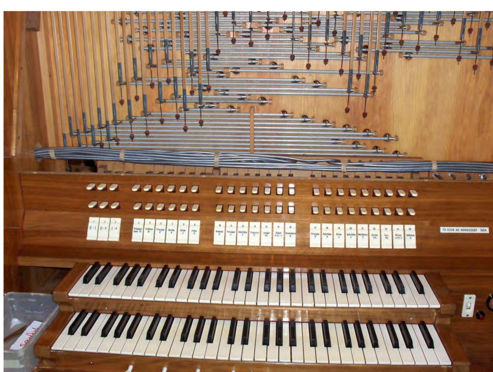
Revision der Orgelfirma Kuhn 2013. Blick auf die zwei Manuale (Tastatur), die Registerschaltung (über der Tastatur) und Wellenbrett (mechanische Übertragung der Tastenbewegung zu den Ventilen, die die Luft zu den Pfeifen verteilen).
