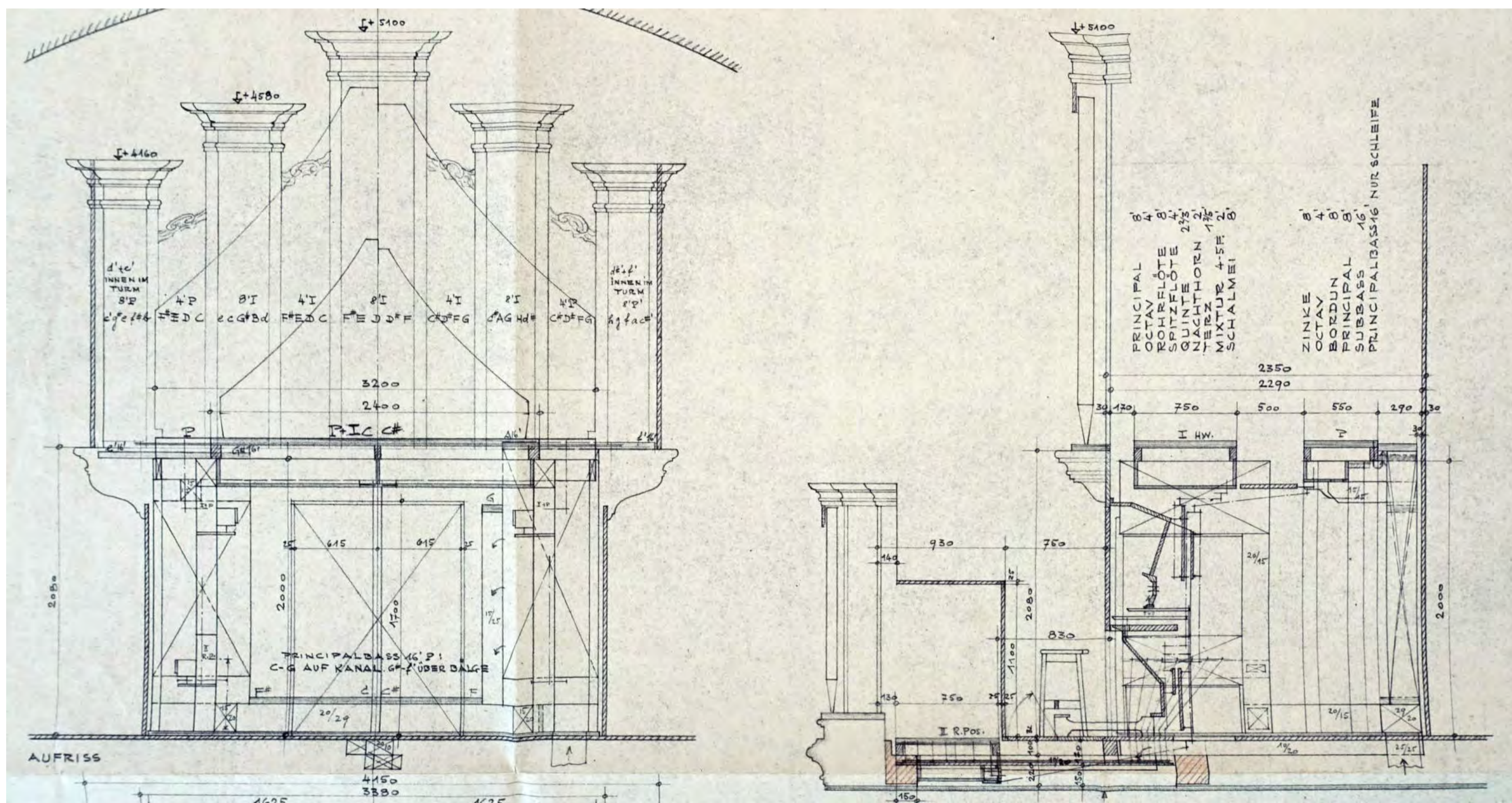
Schnittplan 1:20 der Orgelanlage nach dem Umbau 1954 von Orgelbau Th. Kuhn AG. Links Vorderansicht mit Massangaben und Verteilung der einzelnen Pfeifen. Rechts die Seitenansicht mit Schnitt durch die Orgel.
