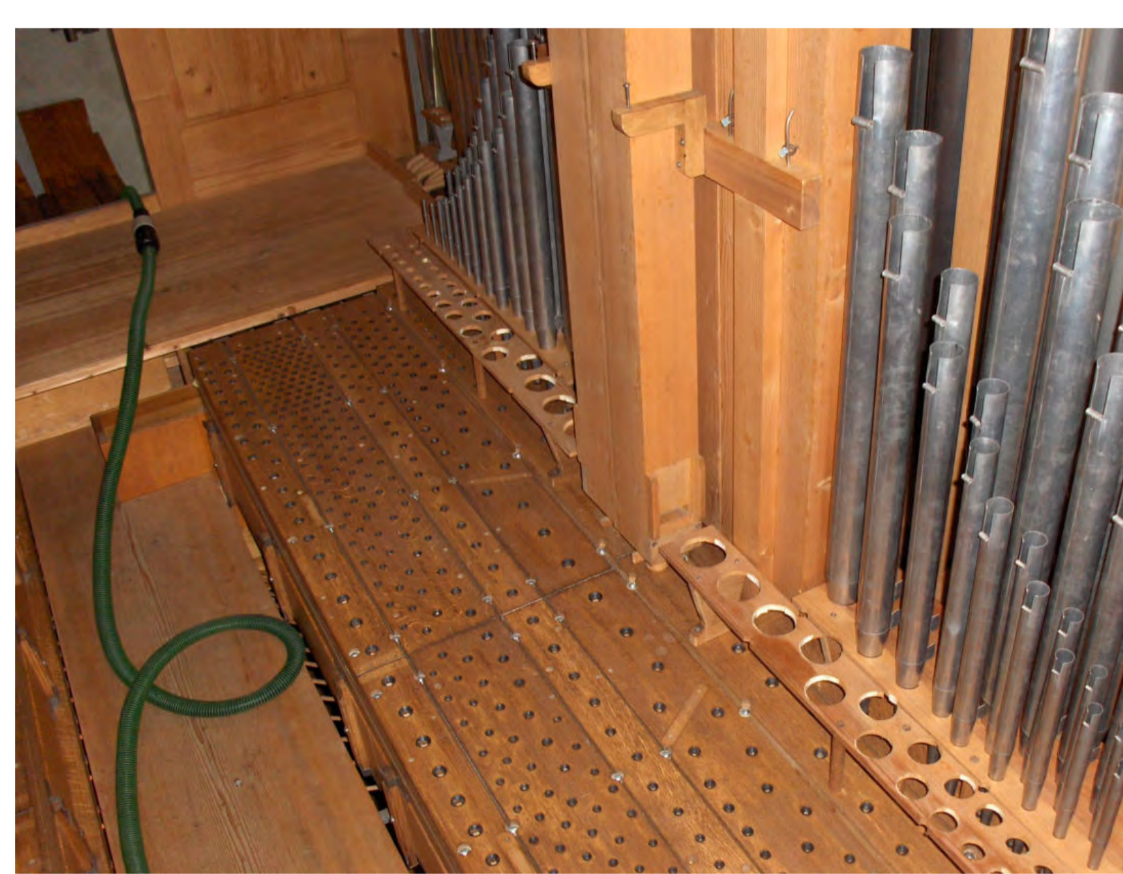
Revision der Orgelfirma Kuhn 2013. Blick auf die Hauptwerks-Windlade (Holzkörper, wo die Luftverteilung zu den darauf stehenden Pfeifen stattfindet).
