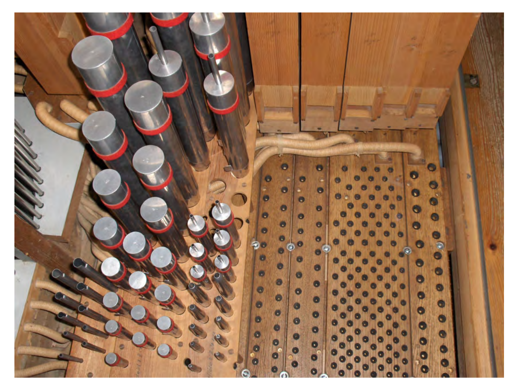
Revision der Orgelfirma Kuhn 2013. Blick auf die Windlade des Rückpositivs. Rückpositiv: Es befindet sich im Rücken des Organisten in einem eigenen Gehäuse und ist in der Emporenbrüstung angebracht.
